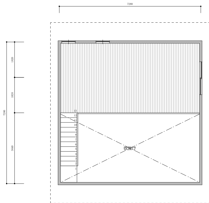
1階平面図
